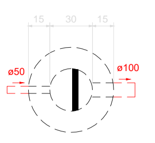
Caixa de gordura - Pavimento Planta baixa - ESC. 1:25
