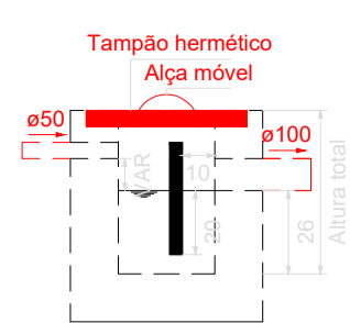
Caixa de gordura - Pavimento Corte 1 - ESC. 1:25
